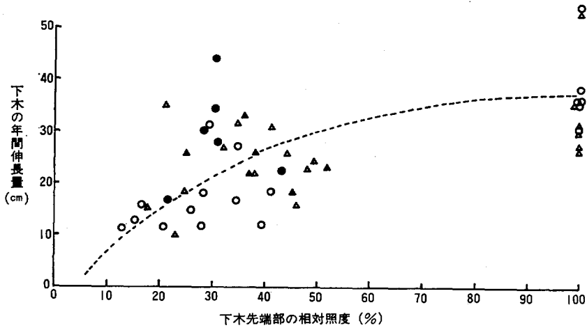
図2. 小田深山試験地の相対照度と下木スギの樹高生長
