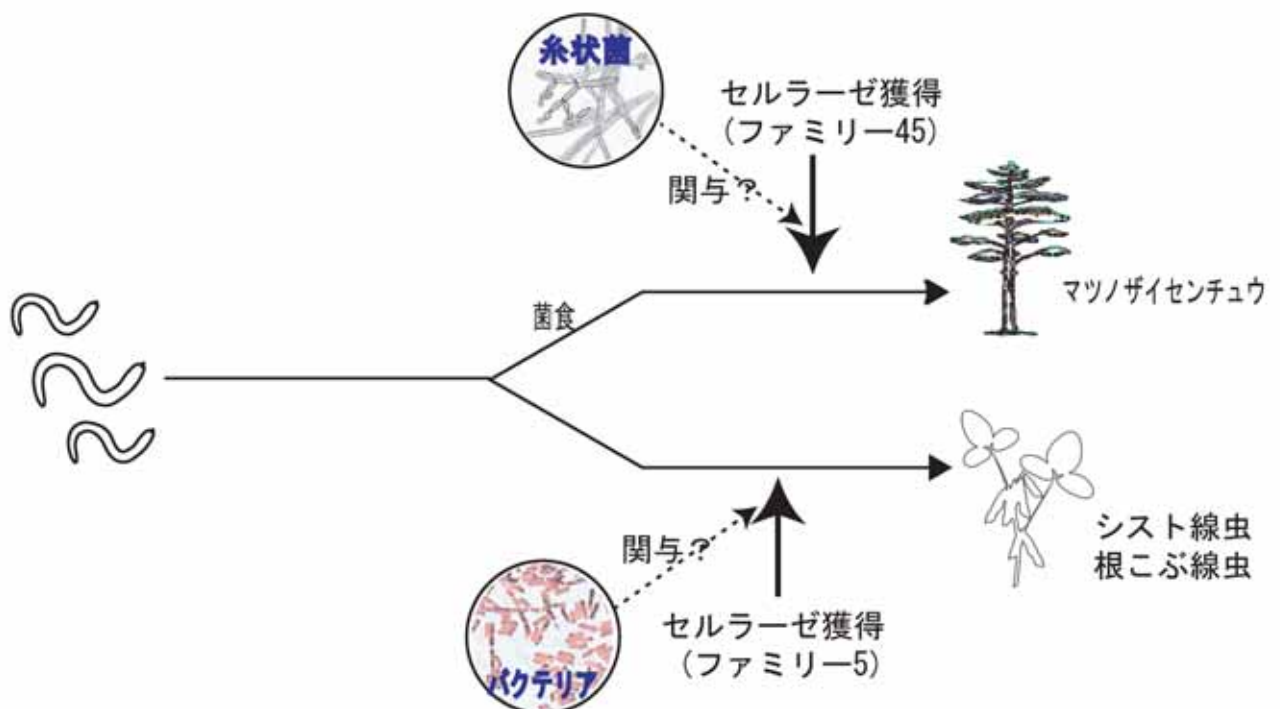
図2. 推定されるマツノザイセンチュウとシスト・根こぶ線虫の植物寄生能力の進化過程
