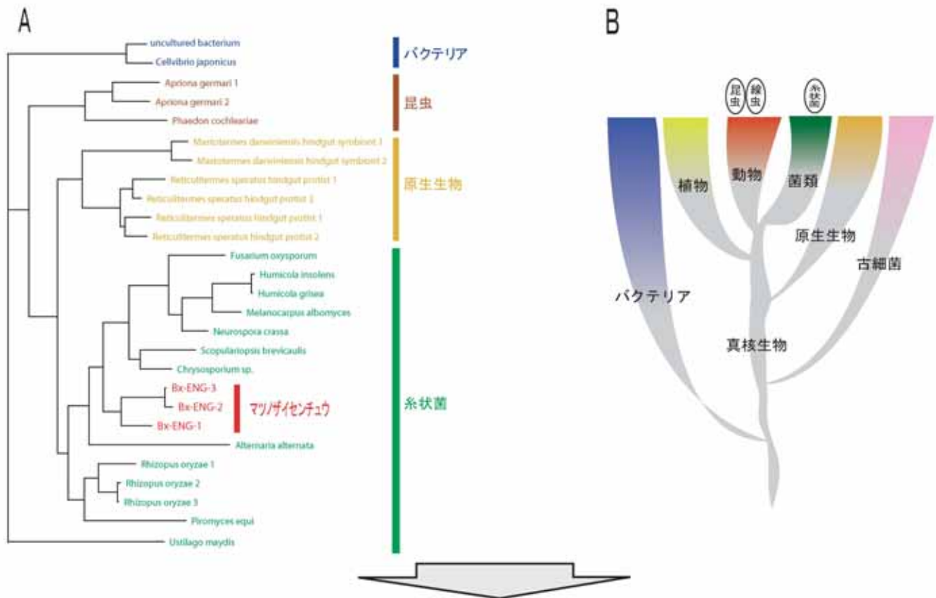
図1. ファミリー45に属するセルラーゼの系統樹(A)と一般的な進化系統樹(B)との比較
