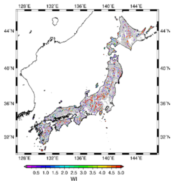
計算期間中の風害リスク示数 (WI) 最大値
