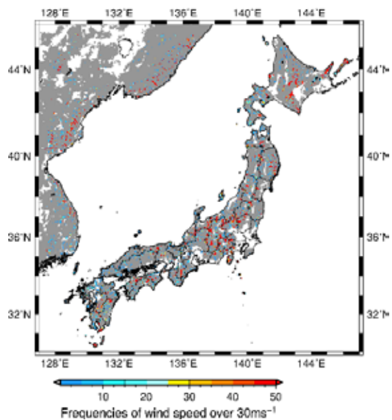
計算期間中の森林域における 風速 30m/s 以上の発生頻度
