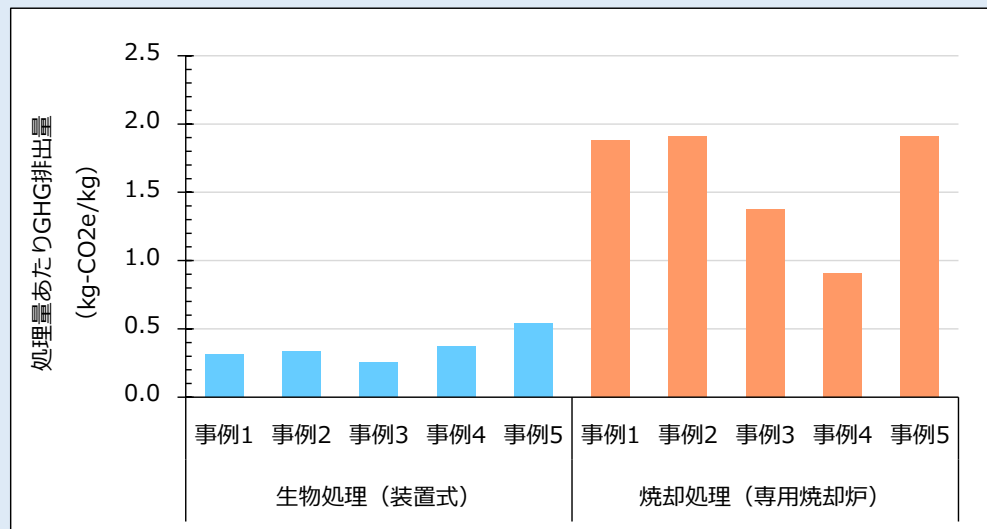
図 処理量あたりの GHG 排出量の試算結果
